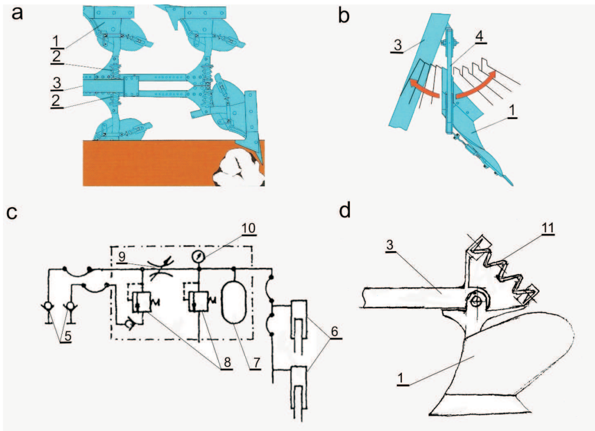
Rys. 7. Wybrane systemy zabezpieczania ram i korpusów płużnych przed przeciążeniem: a) za pomocą „kołka - bezpiecznika”, b) za pomocą sprężystego cięgła (patent firmy Lemken), c) za pomocą układu hydraulicznego, d) sprężynowy (resorowy); 1 - korpus płużny, 2 - ścinowy „kołek bezpiecznik”, 3 - rama, 4 - sprężyste cięgło, 5 - szybkozłącza, 6 - siłowniki nurnikowe, 7 - akumulator hydrauliczno-gazowy, 8 - zawory przelewowe i bezpieczeństwa, 9 - zawór dławiąco-odcinający, 10 - manometr, 11 - sprężyna lub resor
