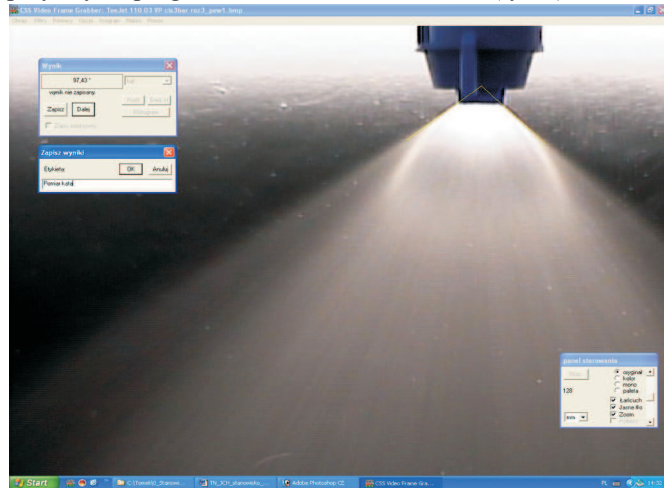
Rys. 2. Widok okna programu MultiScanBase v. 14.02 podczas pomiaru kąta rozpylenia cieczy
