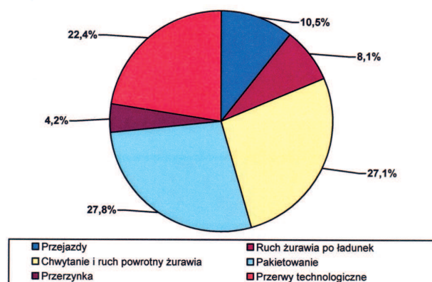
Rys. 3. Struktura cyklu roboczego maszyny do pakietowania pozostałości pozrębowych
