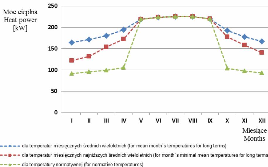
Rys. 3. Nadwyżki mocy cieplnej w gospodarstwie pochodzącej z inwestycji biogazowej obliczone dla różnych temperatur zewnętrznych, przedstawione dla kolejnych miesięcy roku Fig. 3. Heat power surplus in the farm from the biogas-works, calculated for the various external temperatures and presented for the consecutive months of a year
