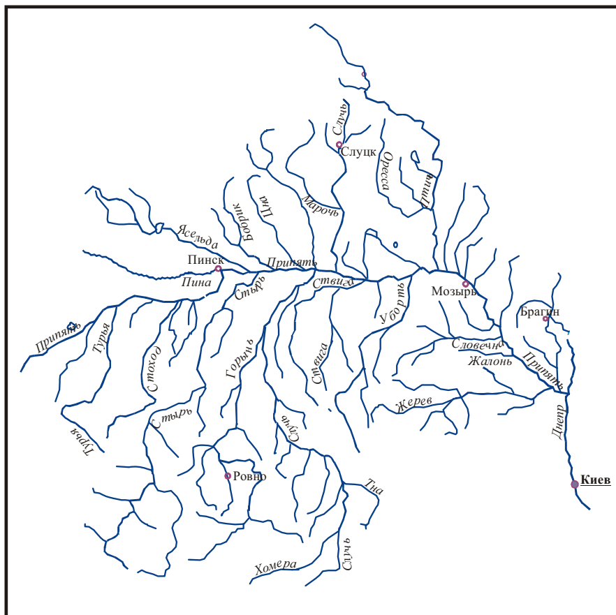
Рис. 1. Гидрографическая сеть бассейна р. Припять Fig. 1. The drainage system of the River Pripet' Basin
