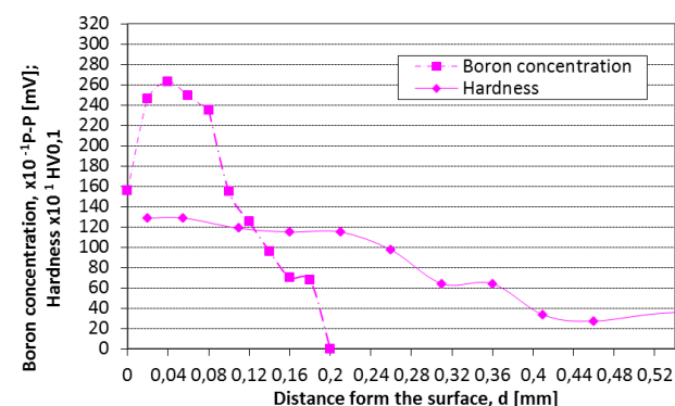
Fig. 6. Change in boron concentration distribution and hardness distribution in the surface layer of nodular iron after laser treatment Rys. 6. Zmiana stężenia boru oraz zmiana twardości w warstwie wierzchniej żeliwa sferoidalnego po obróbce laserowej (opracowanie własne)
