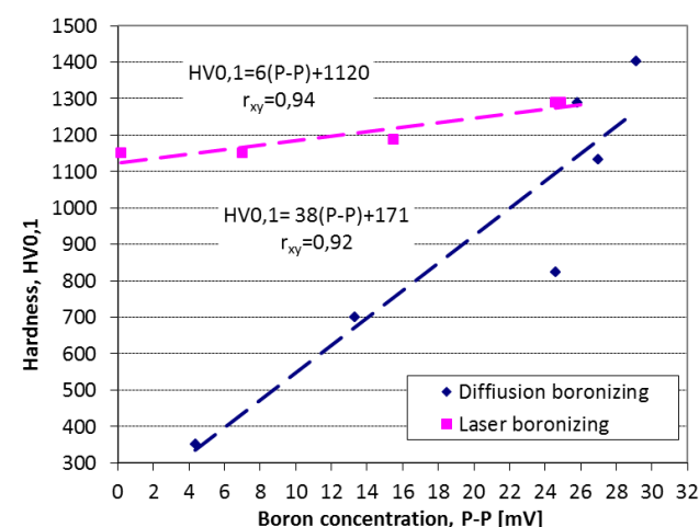
Fig. 7. The correlation between boron concentration and hardness in the surface layer of nodular iron in case of diffusion and laser boronizing Rys. 7. Zależność pomiędzy zawartością boru i twardością w warstwie wierzchniej żeliwa sferoidalnego w przypadku borowania dyfuzyjnego i laserowego
