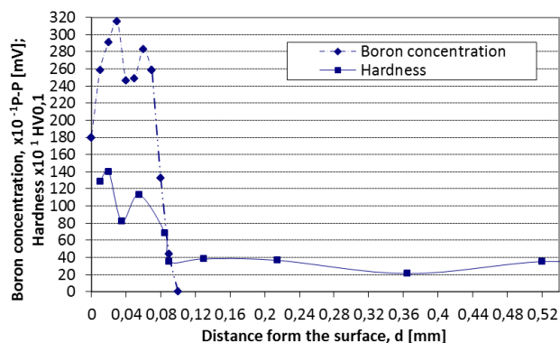
Fig. 5. Change in boron concentration distribution and hardness distribution in the surface layer of nodular iron after diffusion treatment Rys. 5. Zmiany stężenia boru oraz zmiana twardości w warstwie wierzchniej żeliwa sferoidalnego po obróbce dyfuzyjnej (opracowanie własne)
