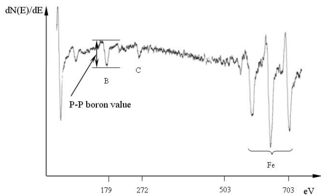
Fig. 4. The example of AES spectrum for the nodular iron surface layer after laser alloying Rys. 4. Przykładowe widmo AES dla warstwy wierzchniej żeliwa sferoidalnego po stopowaniu laserowym
