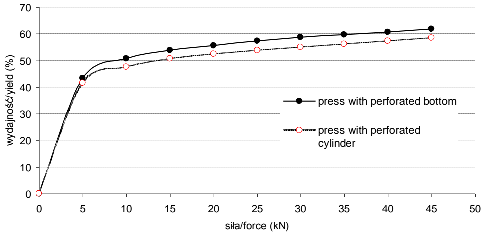
Fig. 3. The effect of applied forces and type of presses on the yield of apple juice Rys. 3. Wpływ siły i rodzaju prasy na wydajność soku jabłkowego
