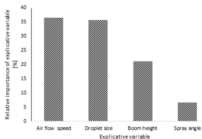
Fig. 4. Effect of independent variables in LPLI model Rys. 4. Wpływ zmiennych niezależnych modelu na W_{so}
