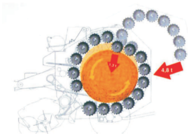
Rys. 2. System maksymalnego zgniotu w prasoowijarce firmy Claas
