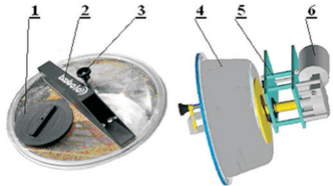
Rys. 1. Budowa modułu Biobolo: 1 - korek wsypu, 2 - rynna dozownika, 3 - śruba dozownika, 4 - obrotowy zbiornik, 5 - uchwyty mocujące, 6 - silnik elektryczny
