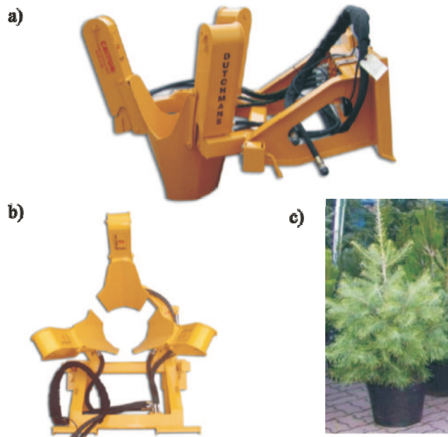
Rys. 5. Przesadzarka wykorzystywana w szkółce zadrzewieniowej Dutchman High Production Field Potter z zamkniętymi łopatami, a - widok z boku, b - widok z góry [www.dutchmantreespade.com], c - sadzonka przesadzona w donicę
