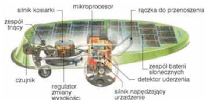
Rys. 2. Schemat budowy kosiarki automatycznej firmy Husqvarna zasilanej energią słoneczną [1] Fig. 2. Diagram of the construction of Husqvarna solar-powered automatic lawn mower [1]
