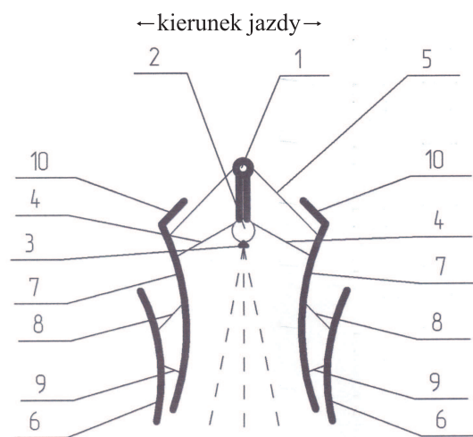
a) osłona dwustronna
