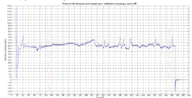
Rys. 5. Wykres momentu obrotowego na wale napędowym dmuchawy przenośnika w czasie załadunku przyczepy - pomiar E1 Fig. 5. Graph of torque on the blower conveyor drive shaft at the time of loading of the trailer - the measurement of E1
