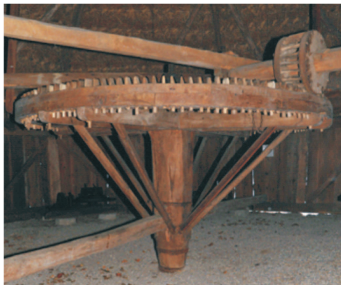
Rys. 8. Kierat z górnym napędem Fig. 8. Horse gear with upper drive
