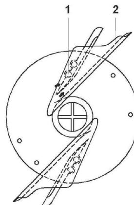
Rys. 2. Tarcza D4 HVXR z podwójnymi łopatkami rozsiewaczy firmy Kuhn [2]: 1 - łopatkę zasilaną nawozem o mniejszym przekroju strumienia, 2 - łopatkę zasilaną nawozem o większym przekroju strumienia
