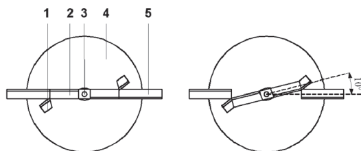
Rys. 4. Tarcze rozsiewaczy Amazone z możliwością zmiany kąta ustawienia łopatek w czasie pracy [3]: 1 - łopatka nawożenia granicznego, 2 - wewnętrzna łopatka obrotowa, 3 - koncentryczny mechanizm ustawczy, 4 - tarcza, 5 - zewnętrzna część łopatki
