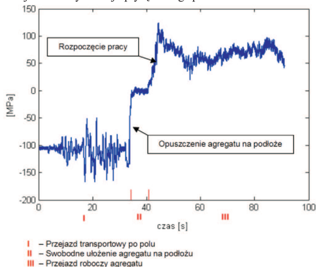
Rys. 6. Przebieg zmian naprężeń w wybranym punkcie pomiarowym
